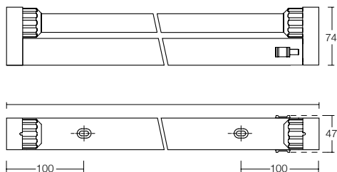
Anschluss über Luxsystem Steckvorrichtung Connection via Luxsystem connector system
