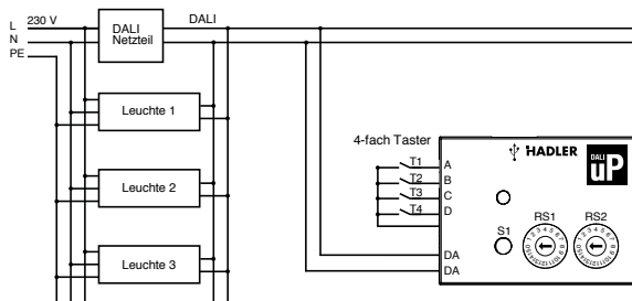
DALI uP Verdrahtungsplan DALI uP wiring diagram
