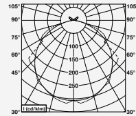
▀ Abdeckung klar (4.200 lm/m bei 3.000 K, < 25 W/m) Cover clear (4.200 lm/m bei 3.000 K, < 25 W/m)
